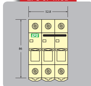
EPS 3P MCB
